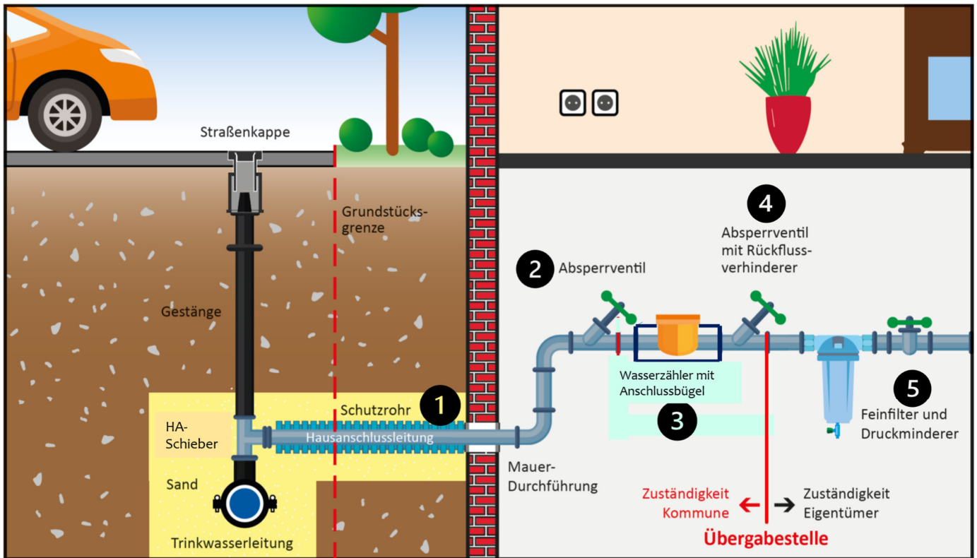
Schemabild
